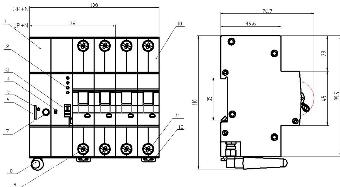
JLIB5LEU-63M3 (100M3) 外形与安装尺寸图
